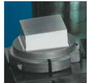
Trumpf oder Amada Halter für Whisper- Anschliff / Trumpf or Amada holders for whisper grinding
