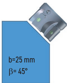
GLW-0715-19-00-00-0 Milling head
